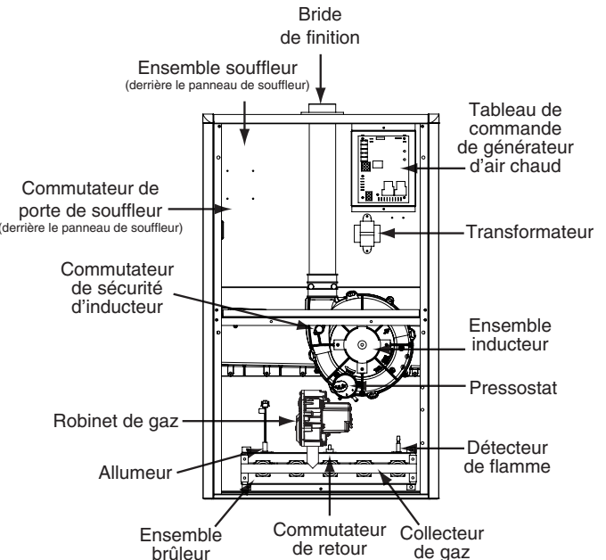
Générateur d'air chaud au gaz à flux descendant à condensation modèles J951X*D
