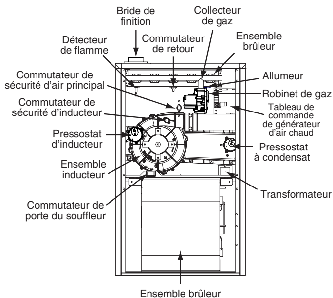
Générateur d'air chaud au gaz à flux ascendant / horizontal à condensation modèles J951X*U
