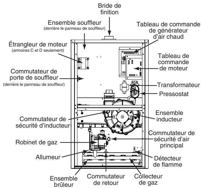
Générateur d'air chaud au gaz à flux descendant à condensation modèles J962V*D
