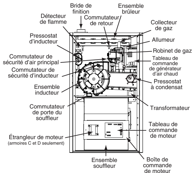
Générateur d'air chaud au gaz à flux ascendant / horizontal à condensation modèles J952V*U
