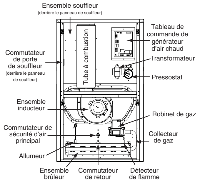
Générateur d'air chaud au gaz à flux descendant sans condensation modèles J801X*D
