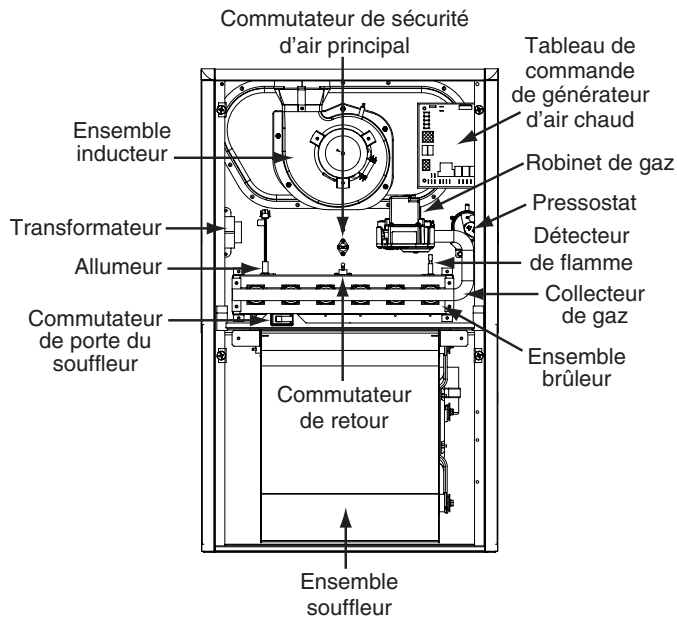
Générateur d'air chaud au gaz à flux ascendant / horizontal sans condensation modèles J801X*U
