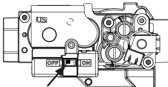
VANNE DEUX ÉTAGES
