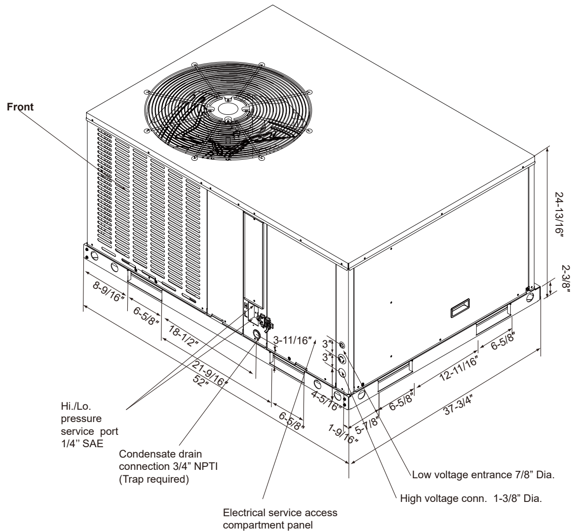
Fig. 2-2 Unit Dimensions
